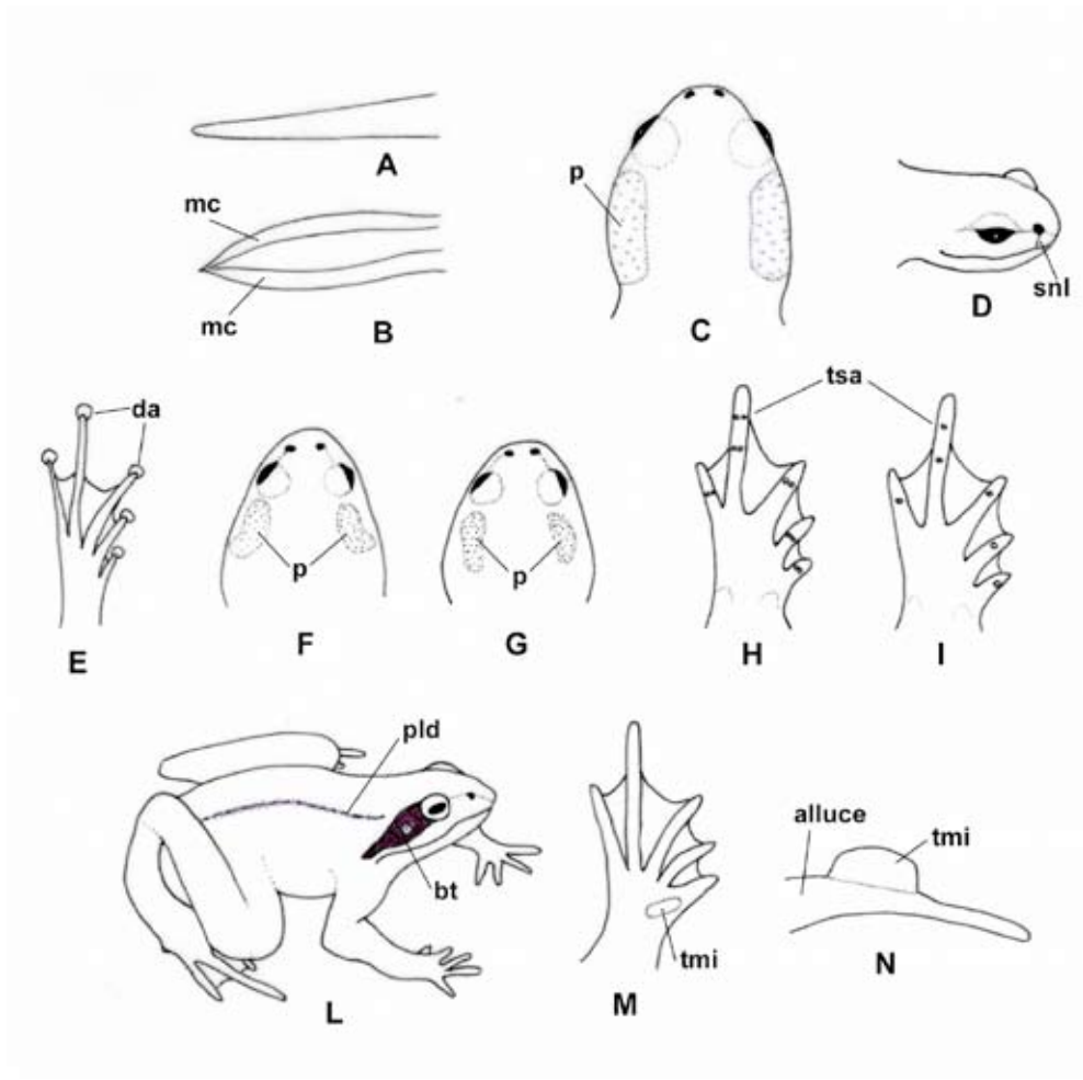
Tav. 1. A: coda di Urodelo a sezione rotonda e senza creste membranose. B: coda di Urodelo a sezione appiattita e con creste membranose (= mc ). C: testa di salamandra pezzata ( p = ghiandola parotoide). D: testa di geotritone ( snl = solco naso-labiale). E: piede di raganella ( da = dischi adesivi). F: testa di rospo comune ( p = ghiandola parotoide). G: testa di rospo smeraldino ( p = ghiandola parotoide). H: piede di rospo comune, dal lato ventrale ( tsa = tubercoli sotto-articolari). I: piede di rospo smeraldino, dal lato ventrale ( tsa = tubercoli sottoarticolari). L: esemplare del genere Rana ( bt = banda temporale; pld = pliche latero-dorsali). M: piede di rana, dal lato ventrale ( tmi = tubercolo metatarsale interno). N: alluce di rana di Lessona, in visione laterale ( tmi = tubercolo metatarsale interno) [le figg. H, I, M e N da LANZA, 1983, ridisegnate e modificate].
